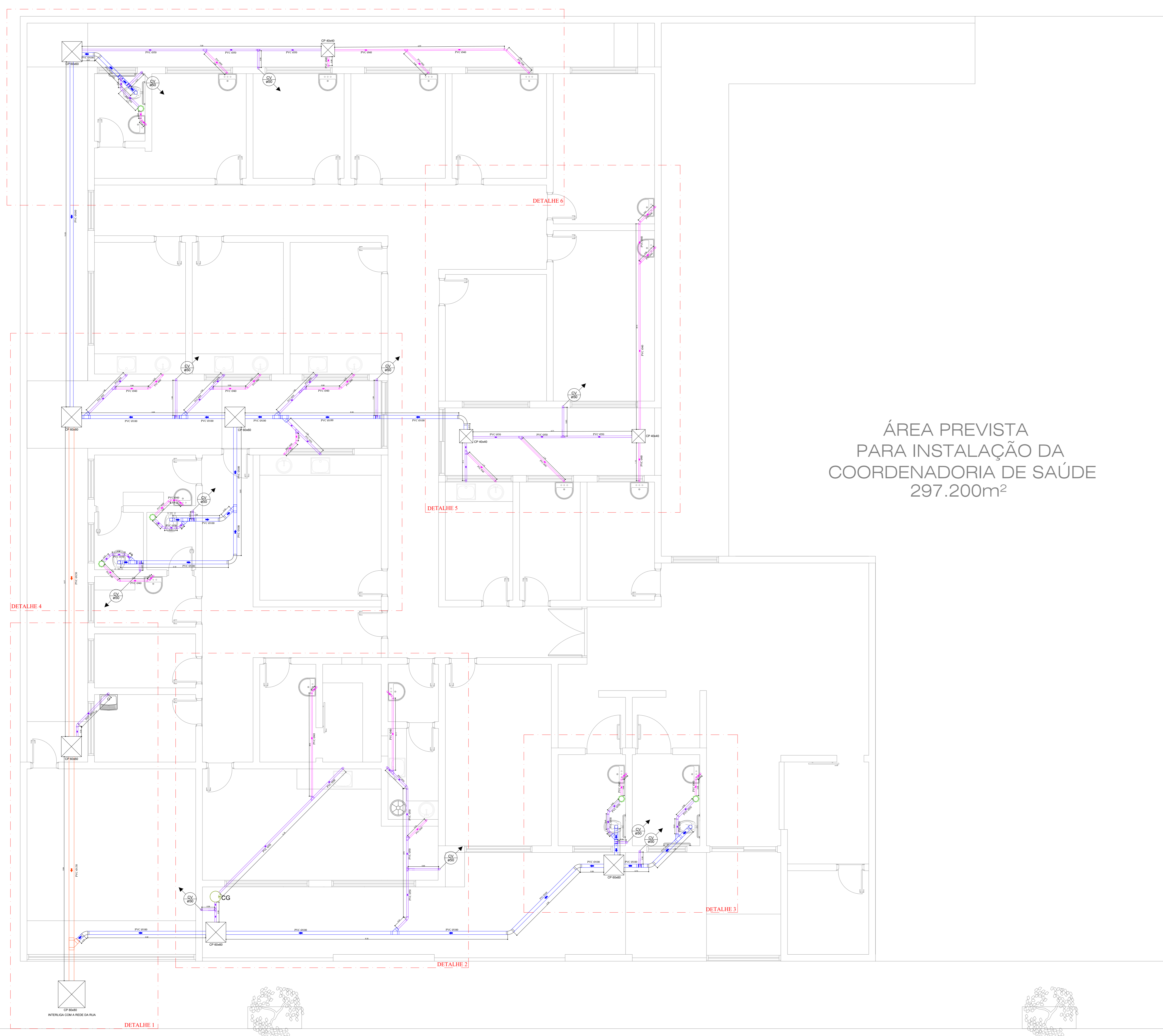
PLANTA BAIXA - ESGOTO SANITÁRIO Escala 1:50
